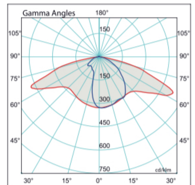
Işık Şiddeti Dağılım Eğrisi Light Distribution Curve
