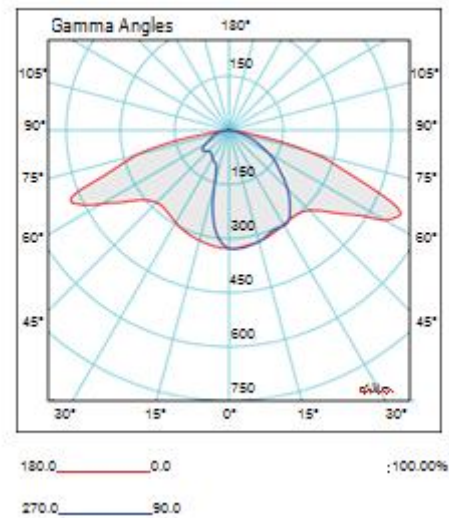
Işık Şiddeti Dağılım Eğrisi Light Distribution Curve
